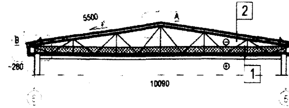
GRIEZUMS 1-1, M 1:200
